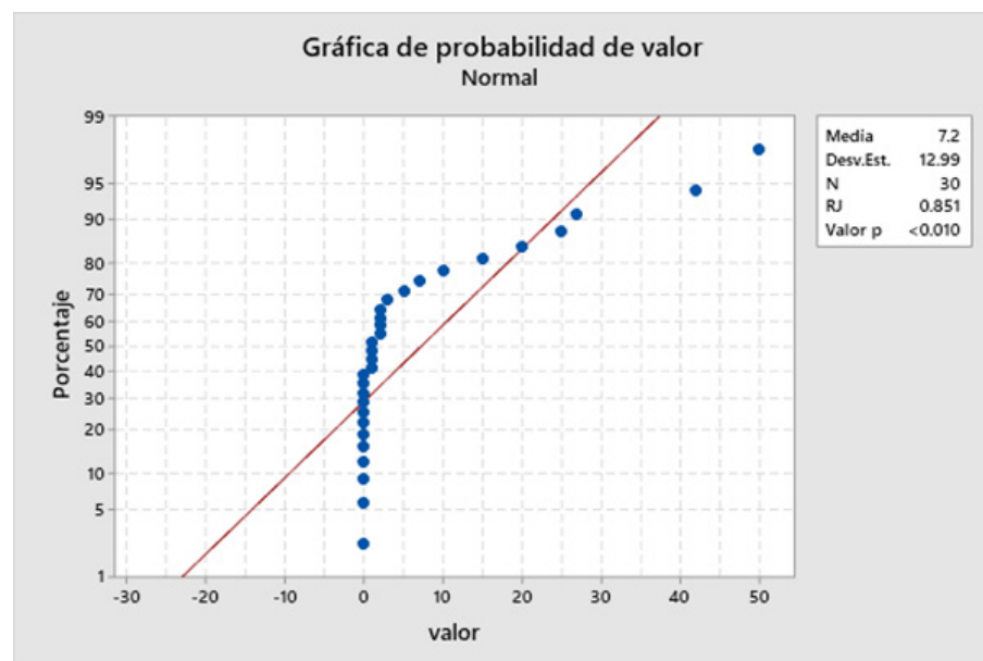
Resultados de prueba de normalidad de distribución de los datos
